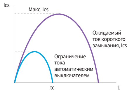
Характеристика ограничения тока
