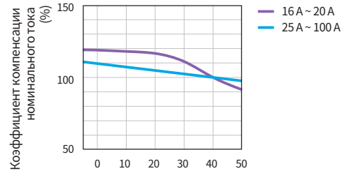
График снижения номиналов по температуре
