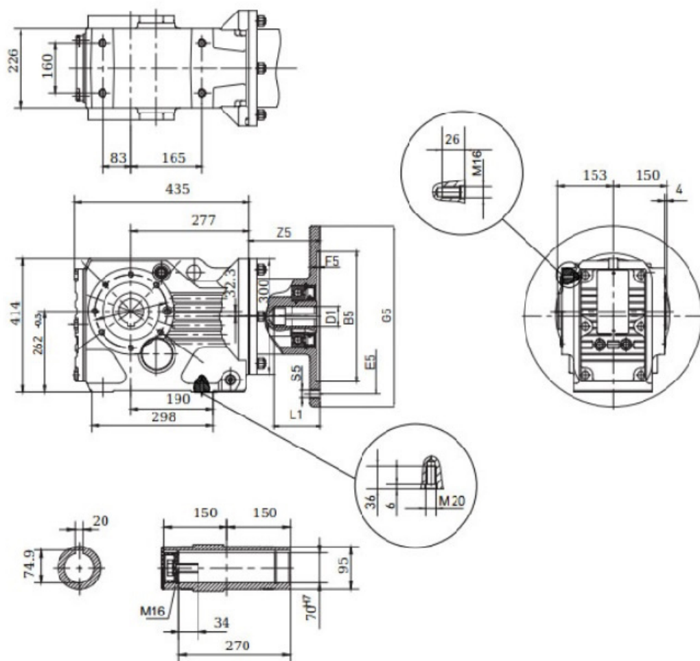
Размеры входного фланца для присоединения двигателя
